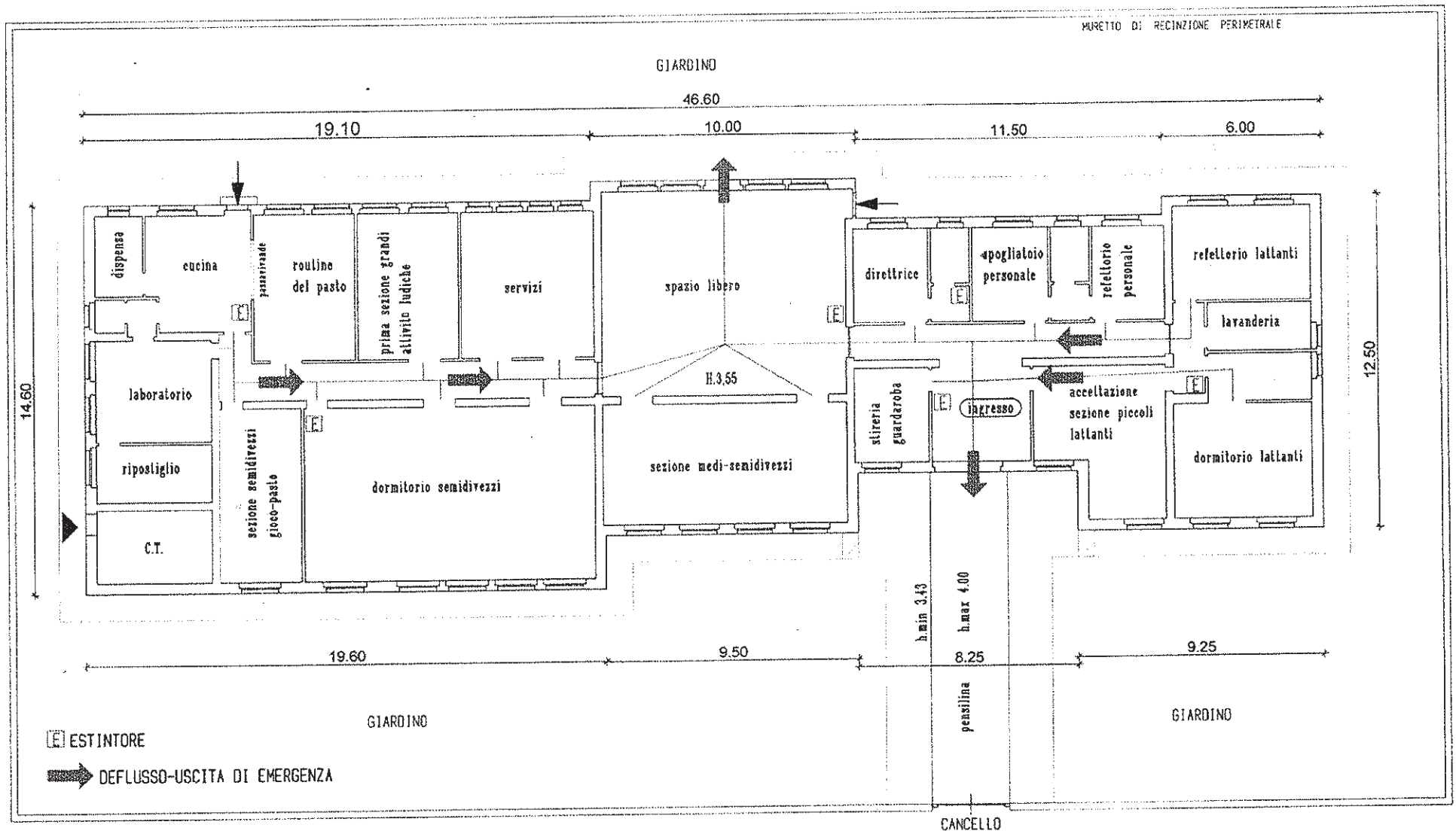
PLANIMETRIA DI EMERGENZA - PIANO TERRA- ASILO NIDO A. GRAMSCI - ORTONA (CH)
