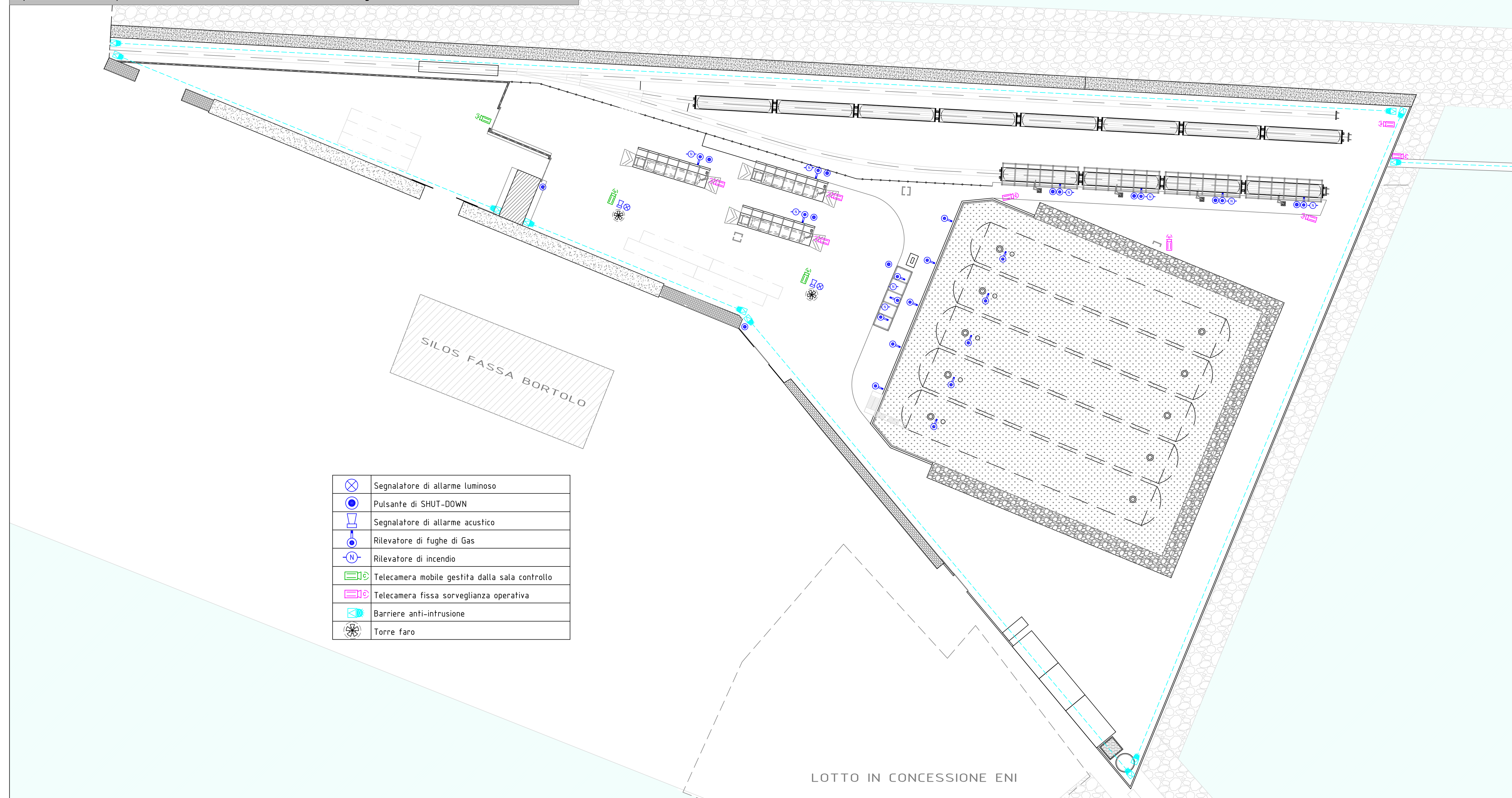
Impianto di TVCC, impianto anti-intrusione, rilevazione e rivelazione gas e incendio - DEPOSITO- (scala 1:500)
